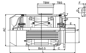
IM B35 Kivitel 2
