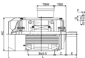
IM B3 Kivitel 1
